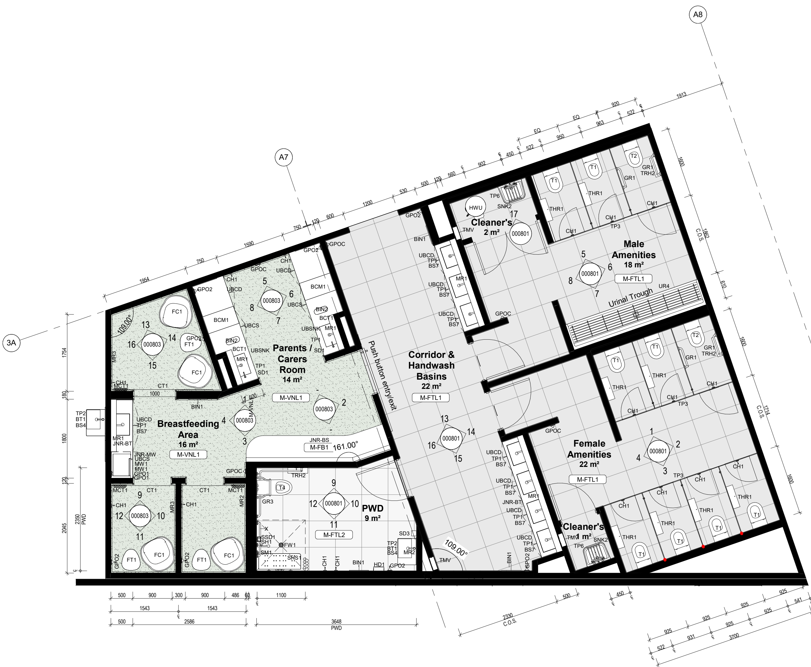
1 WET AREA PLAN - Area 51 1 : 50
